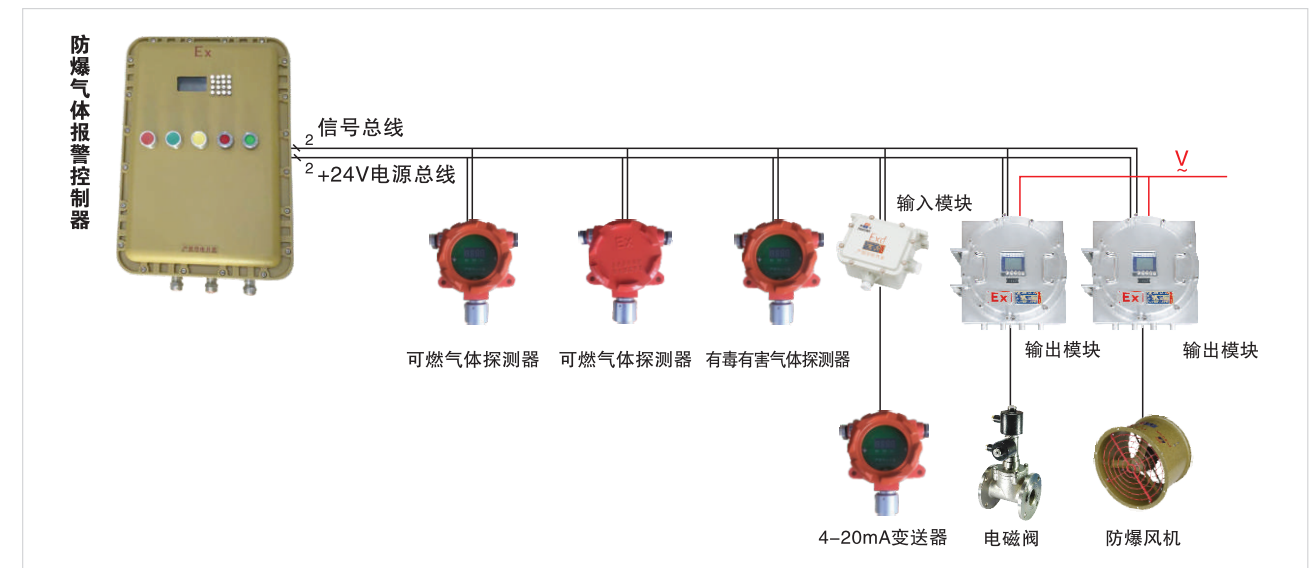
腾达防爆科技固定式气体检测报警仪示意图
