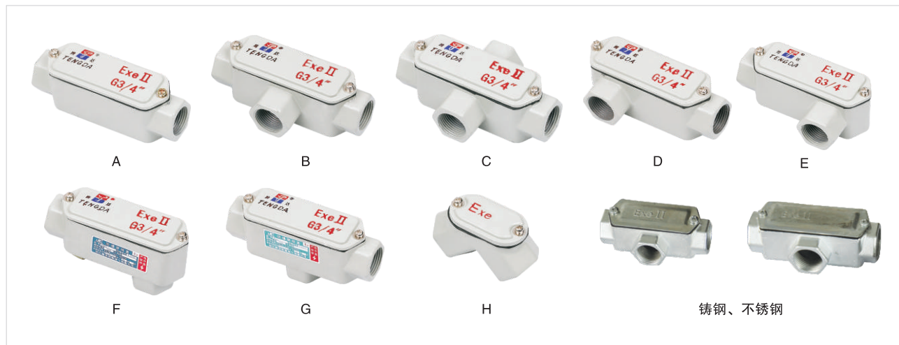
BHC系列防爆穿线盒(e)
